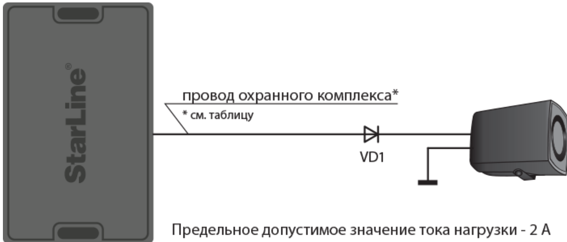
Схема подключения автомобильной сирены
